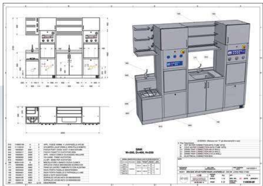
Schema installazione di un locale chiavi in mano AT-OS.
